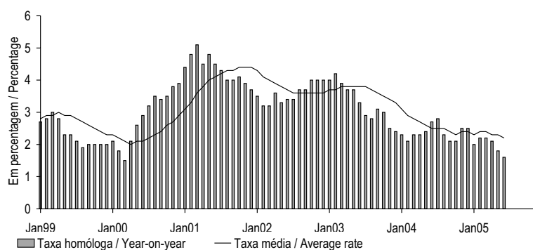
IPC/CPI
