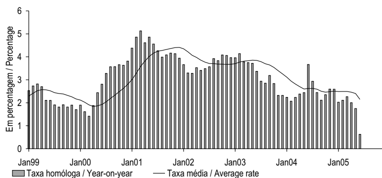
IHPC/HICP
