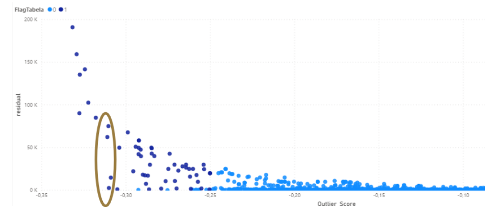
Identificação de outliers no reporte da CRC (2020)
