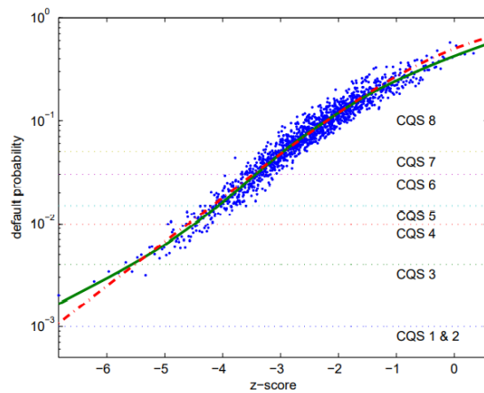
Probabilidade de incumprimento de empresas não financeiras em Portugal (2016)
