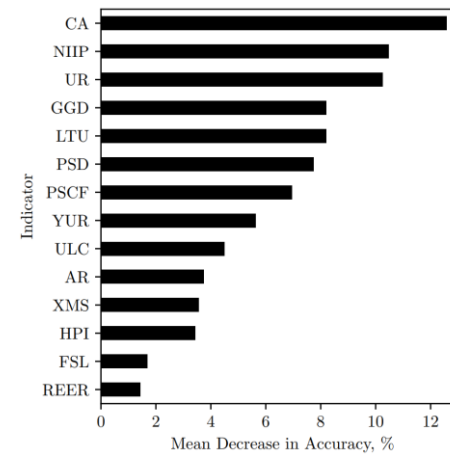
Variáveis mais relevantes do Procedimento de Desequilíbrios Macroeconómicos da UE (2020)
